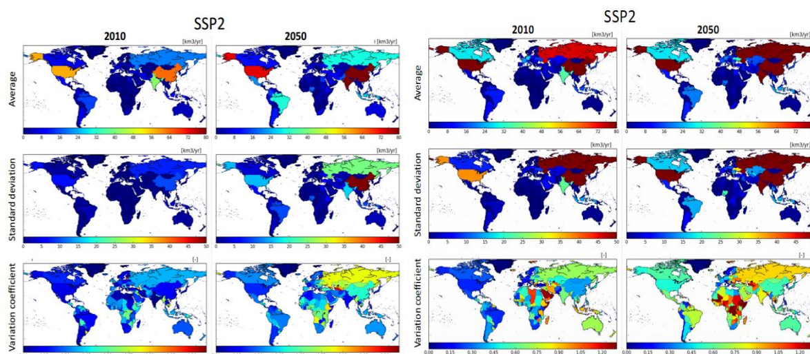
图 2 基准情景下 2010、2050 年全球水资源需求量（左图为家庭生活需水、右图为工业需水） （唐霞 供稿）
