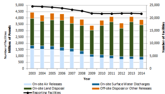
图 1 2003-2014 年 TRI 设施管理的废弃物图 2 2003-2014 年排放的有毒物质
